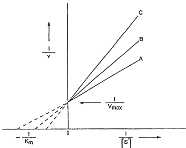
Kompetiční inhibice podle Lineweaverova-Burkova grafu: A – normální neinhibovaná reakce B a C – dvě různé koncentrace inhibitoru (B<C)
