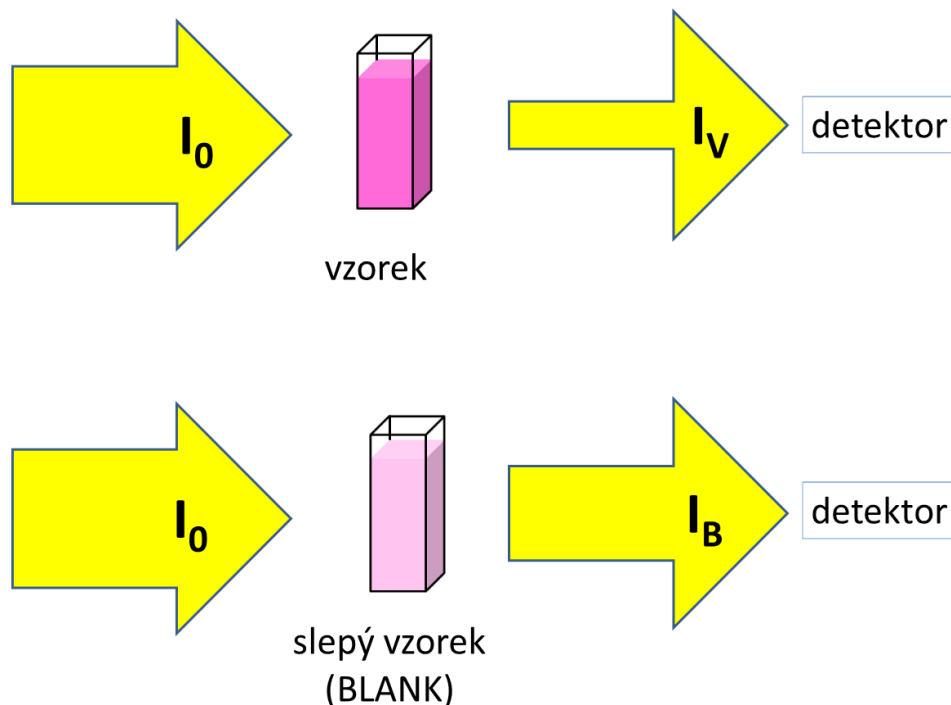
Princip měření absorpčním spektrofotometrem
