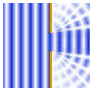
Difrakce malé štěrbině
