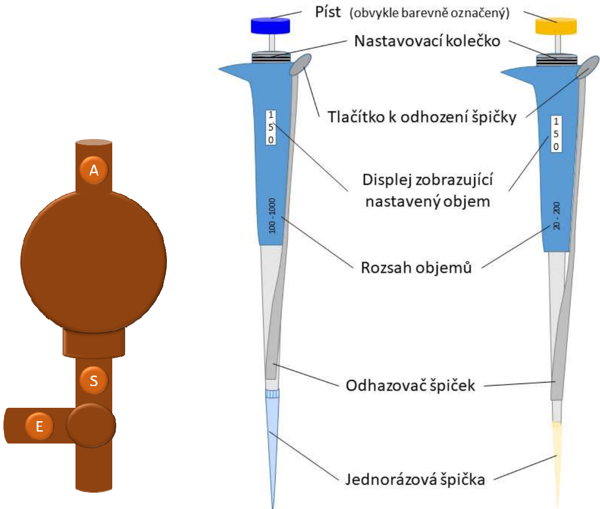
Pipetovací balónek
