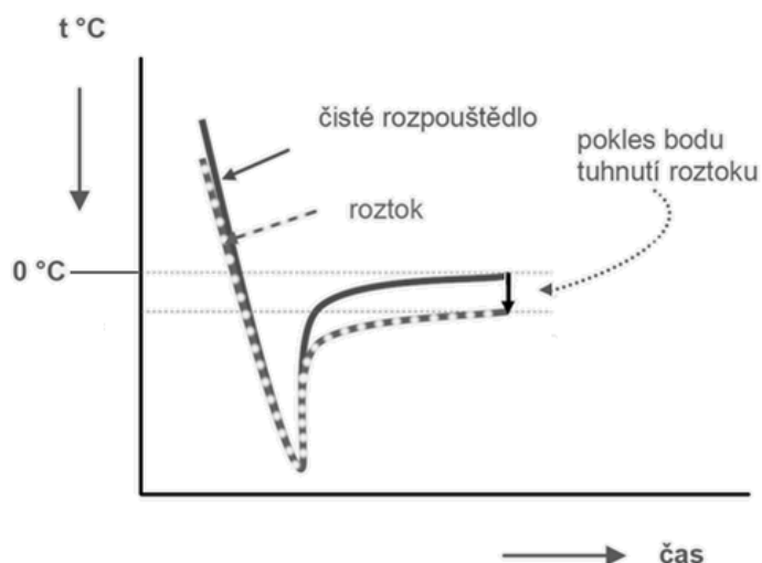
Grafické vyjádření průběhu teplotních změn při kryoskopii
