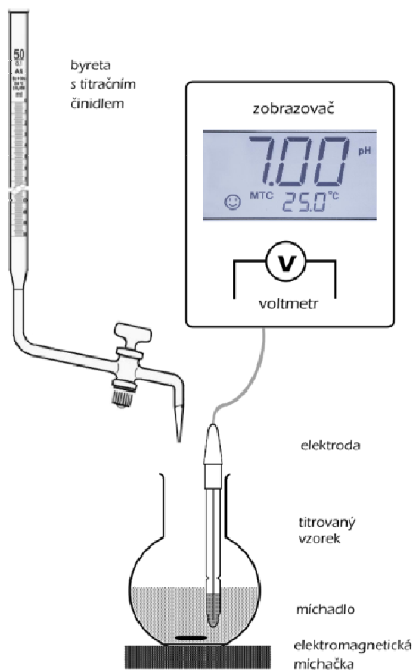
Potenciometrická titrace
